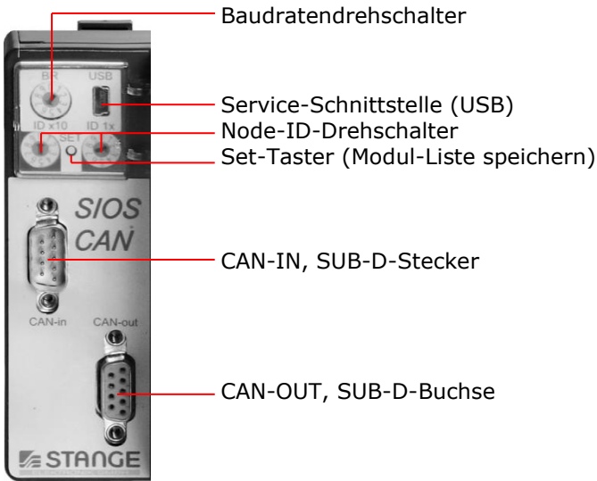
Abbildung 1; Gateway
