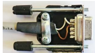
Abbildung 4; CAN-Leitung SE-Gerät <-> SIOS-Gateway
