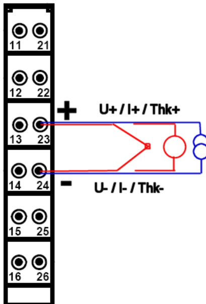
Abbildung 11; IW1-XL-Modul Anschlussbelegung
