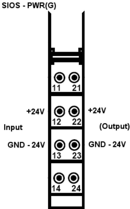
Abbildung 8; PWR-Modul Anschlussbelegung
